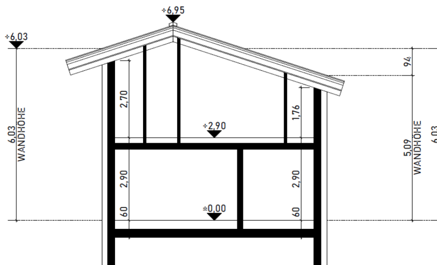
Schnitt Haustyp A
