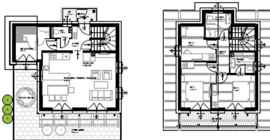
Konzeptgrundriss Haustyp B
